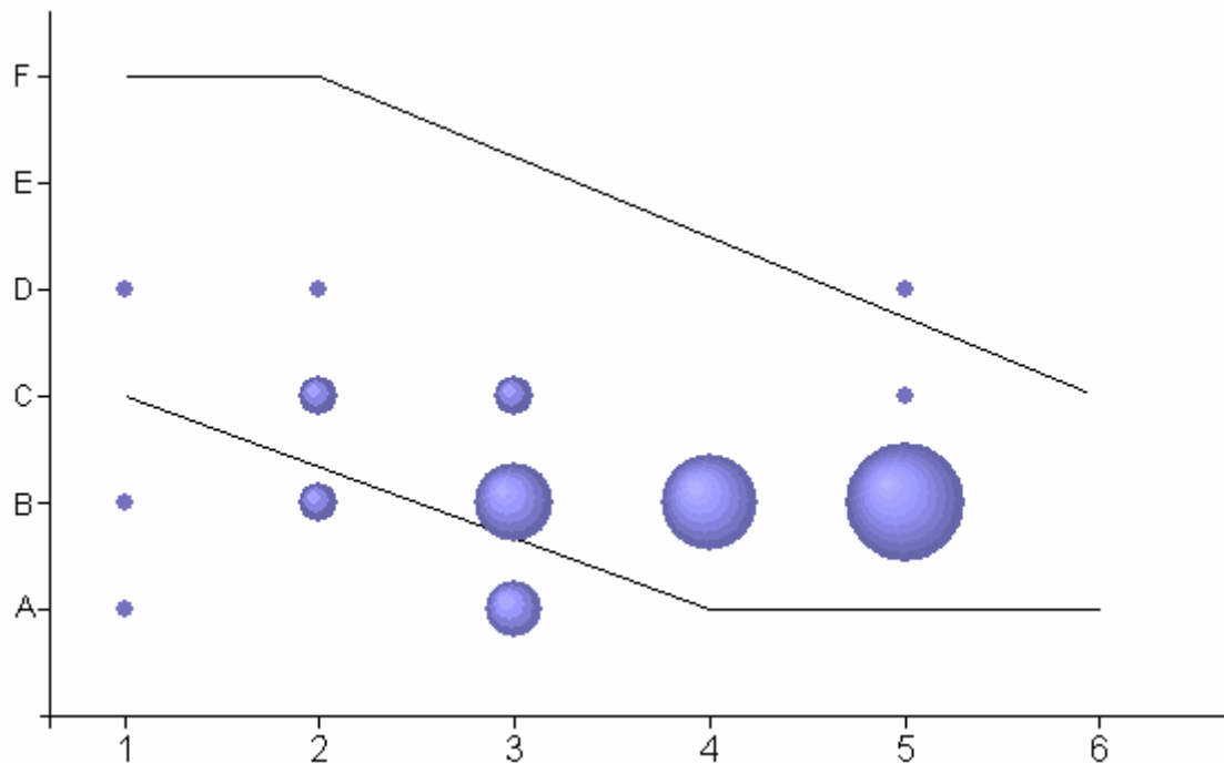
Abbildung 3: Bewertung der Fehler- und Einflußmöglichkeiten nach Durchführung aller Maßnahmen
